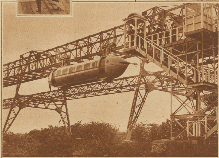
Die neue Hochbahn von Milngavie. Die 20 Personen fassenden Kabinen haben das Aussehen eines Luftschiffes
