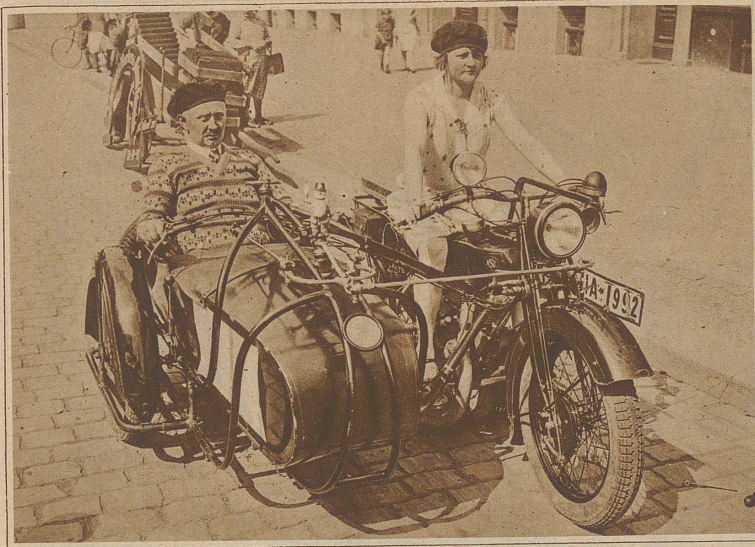
Ein neuartiges Motorrad ist von einem Berliner Fachlehrer konstruiert worden. Es kann vom Seitenwagen aus gesteuert und gefahren werden. Alle Handgriffe des Fahrers auf dem Motorrad werden automatisch auf die Beiwagen-Steuerung übertragen und der Fahrlehrer hat so seinen Schüler immer in seiner Gewalt
