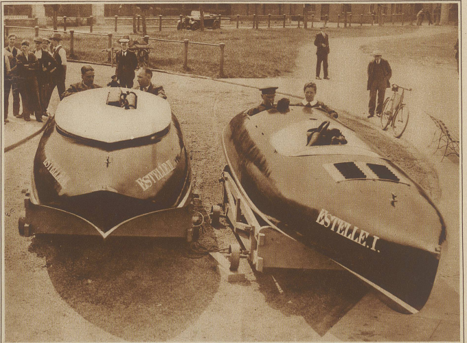
Miss Carstairs, eine junge reiche Engländerin, hat sich ingeheim zwei Motor-boote (Estelle I und II) bauen lassen, die beide mit 1000-erzigen Motoren aus-gerüstet sind. Sie will damit im Monat Juli den Atlantischen Ozean überqueren u. hofft New York in weniger als 3 Tagen zu erreichen. Die Boote erreichen eine maximale Stundengeschwindigkeit von 100 km. Miss Carstairs sitzt am Steuer von Estelle I
