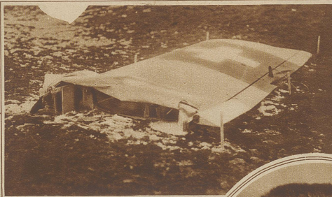
Die während des Fluges gebrochene Tragfläche, die etwa 1 km von der Absturzstelle entfernt gefunden wurde
