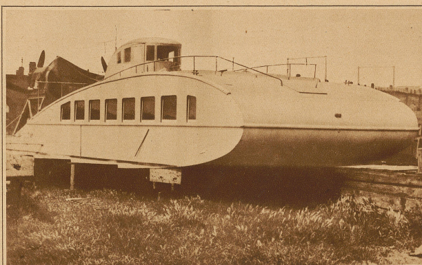
Eine neuartige Schiffsconstruction. In Wien wurde kürzlich das erste Gleitboot für den Donauverkehr von Stapel gelassen. Man rechnet allgemein damit, daß dieses eigenartig gebaute Schiffchen gute Dienste leisten wird
