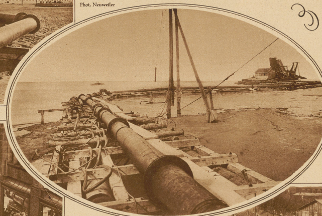
Planierungsarbeiten vor den Flughallen bei Altenrhein am Bodensee. Phot. Neuweiler
