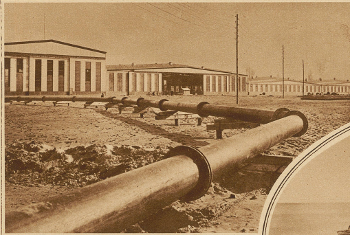
Blick auf die Flughallen. Im Vordergrund ein Teilstück der 1000 Meter langen Rohrleitung, durch welche der Seeschlamm auf das Flugfeld geschwemmt wird.
