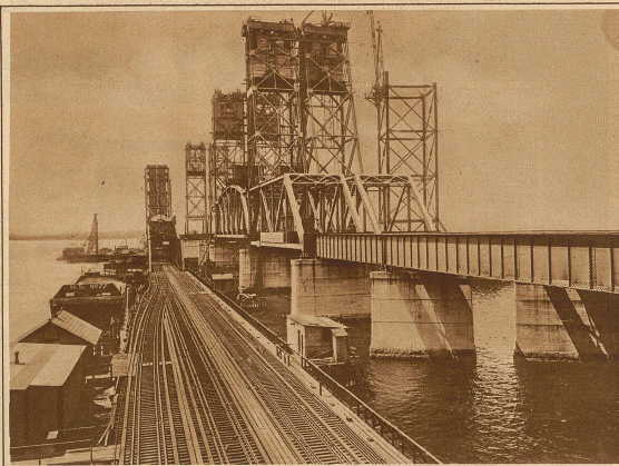
Das Mittelstück mit der Aufzugsvorrichtung
