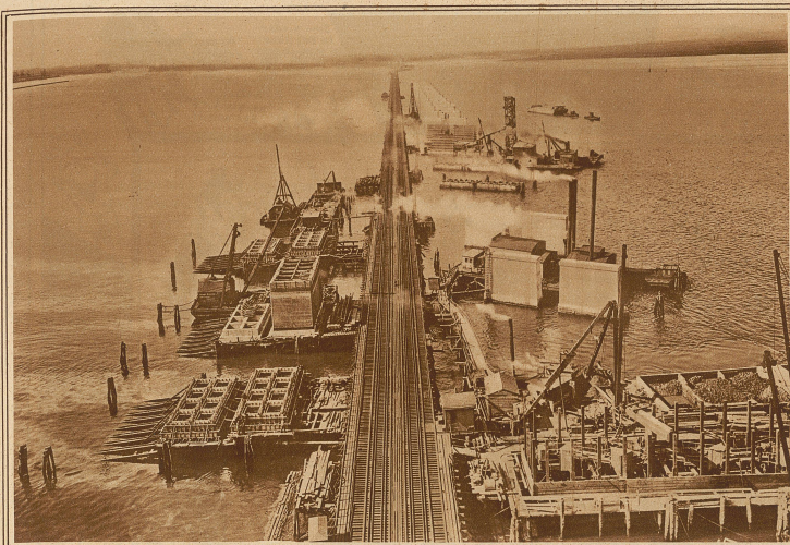
Teilansicht der Brücke während des Baues
