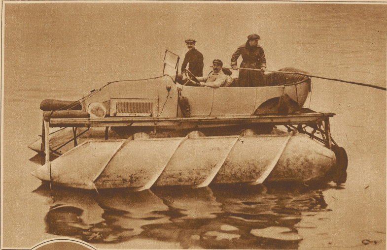
Ein neuer Typ eines Motorbootes, das seine ersten Versuchsfahrten auf der Seine machte. Die Vorwärtsbewegung erfolgt durch die Rotation der Schwimmer
