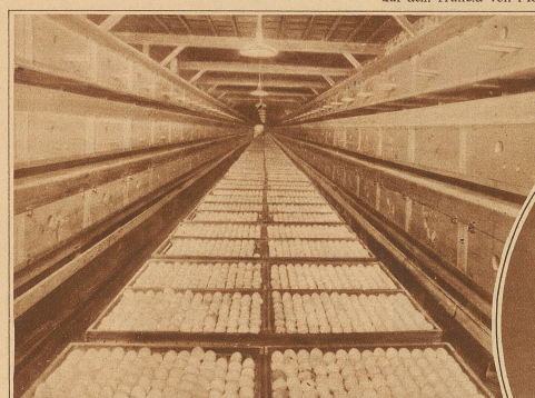
Blick in eine Hühnerbrutanstalt in Petaluma (Kalifornien), die gänzlich mit Elektrizität betrieben wird und in der täglich 50000 Hühner auszubrüten. Von der Anstalt aus werden die Hühner per Eisenbahn und per Schiff in alle Staaten befördert
