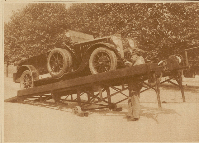
Das Autodock, eine wichtige Erfindung für Automobilisten. Seine Konstruktion erlaubt auch die bequeme Ausführung solcher Reparaturen, die früher nur auf dem Rücken liegend vorgenommen werden konnten
