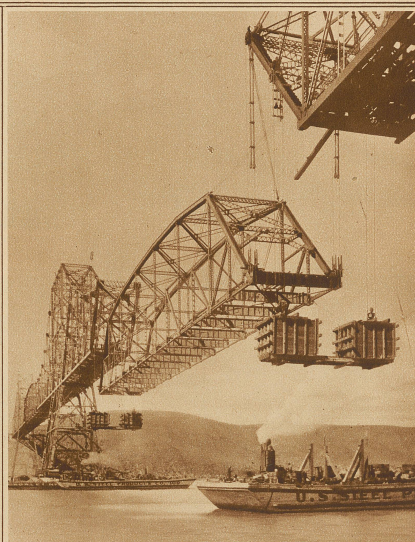
Die Gewalt der Technik. Die neue Eisenbahnbrücke über die Carquinez «Streets» an der San Francisco Bay, die jetzt ihrer Vollendung entgegengeht. Unser Bild zeigt das Einfügen des Mittelstückes
