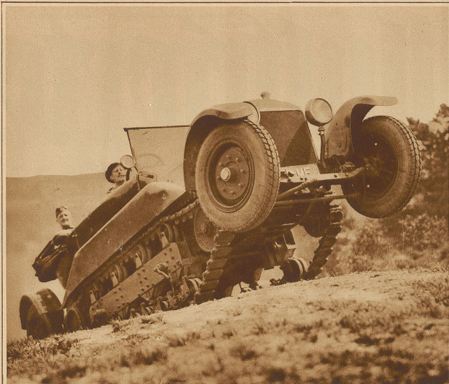
Das neueste Motorfahrzeug stellt eine sinnvolle Kombination von Automobil und Raupenwagen dar. Auf schlechtem Terrain werden die Automobillräder hochgeschaltet. Kehrt das Fahrzeug auf die Straße zurück, so genügt ein Hebelgriff, um es wieder als gewöhnliches Auto fahrbereit zu machen
