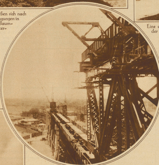
Die größte Hängebrücke der Welt wird gegenwärtig im Hafen von Sydney (Australien) gebaut. Ihre Gesamtlänge wird nach Fertigstellung über 1200 m betragen und die Baukosten belaufen sich auf 125 Millionen Franken
