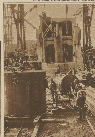
Die Versenkung des Mägelertunnels bei Friedrichshagen, der über Wasser vollständig fertiggestellt und dann als Fußgänger-tunnel in den Fluß versenkt wurde
