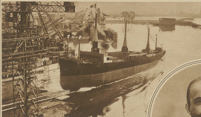
Stapelplatz eines neuen Rennschiffes. Auf der 'Westworth' in Bremen lief letzte Woche das neue, 300 Tonnen große Rennschiff 'Barbar' von Stapel. Es ist das größte bisher gebaute Schiff, das einzig durch den Druck der rotierenden Luftschrauben vorwärts be- wegt wird.
