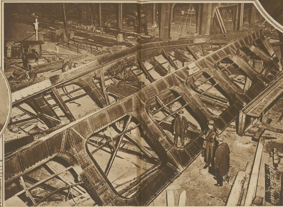
Der eingestürzte Laufkran des Kraftwerkes Rummelsburg.
