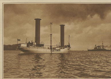
Zur Amerikafahrt des ersten Flettner-Rotor-Schiffes. Das Rotor-Schiff passiert bei seiner Ausfahrt aus dem Kieler Hafen das deutsche Linienschiff „Hessen“.
