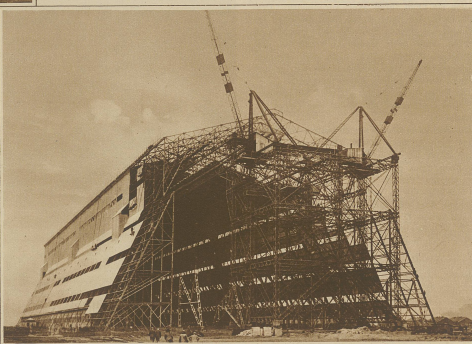
Die größte Luftschiffhalle der Welt wird gegenwärtig auf dem Flugfeld von Cardington (England) gebaut. Sie soll zur Aufnahme der riesigen Passagierluftschiffe dienen, die sich gegenwärtig in England im Bau befinden.
