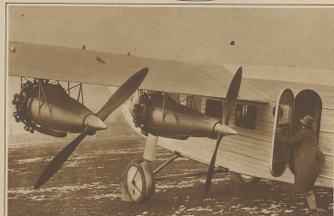
Ein neues deutsches Gredowkehrflugzeug aus den Udetwerken. Wie im Bilde ersichtlich, besitzt der Apparat beidseitig je zwei Motoren, die größte Betriebssicherheit garantieren sollen
