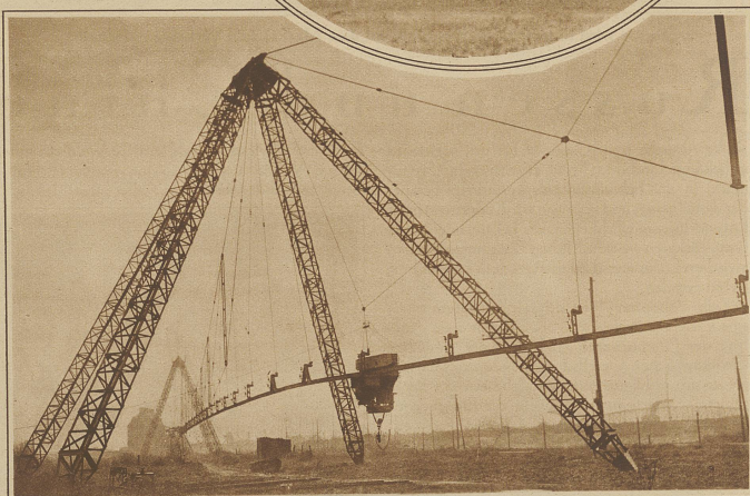
Bei Hamburg ist eine Versuchsbahn zur Beförderung von Lastkähnen erbaut worden. Die Kähne werden durch einen auf einer Schwebeschiene laufenden Motor gezogen.
