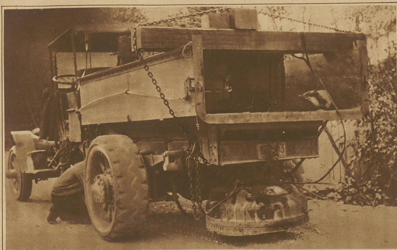
Magnetische Reinigung von Automobilstraßen. In Amerika werden zur Reinigung von Automobilstraßen große Laster, unter denen ein riesenmagnet angebracht ist, verwendet. Der Magnet besitzt ungefähr 250 Volt und zieht sämtliche Eisenteile, Nägel usw. im Umkreis von einem Meter an. Unser Bild zeigt das Magnet-Straßenreinigungs-Auto im Betrieb
