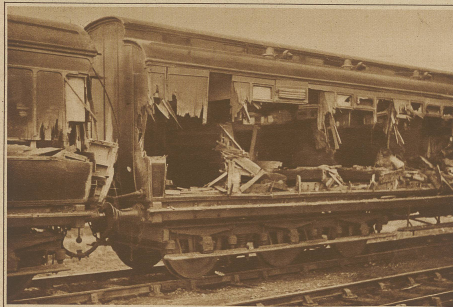
Ein eigenartiges Eisenbahnunglück ereignet sich in Parkgate bei Rotherham (England). Im Augenblick, als die L. M. S. Express mit 80 km Geschwindigkeit einen Cliverton kreuzte, sprang der letzte freie Schienenwagen aus den Schienen und riss an zwei Wagen des vorbeisauenden Expresses die Seitenwände heraus, wobei 9 an den Enden stehende Personen getötet wurden
