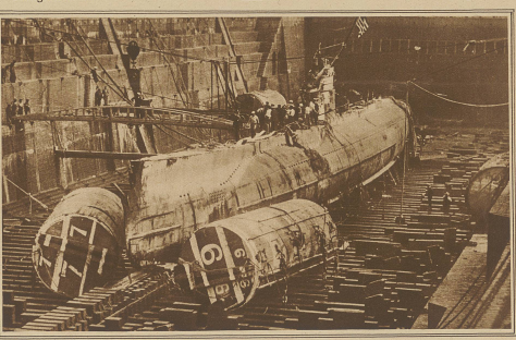
Das amerikanische U-Boot S-51, das vor einem halben Jahr gerammt wurde und mit Mann und Maus unterging, konnte gehoben werden und liegt nun auf dem Trockendock des Newyorker Hafens
