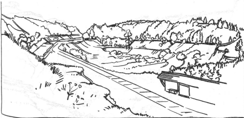
Fig. 4. Höwennegg. Durch die Basaltausbeutung freigelegte Kratertuffmulde, die vordem mit kompaktem Basalt angefüllt war. 1
