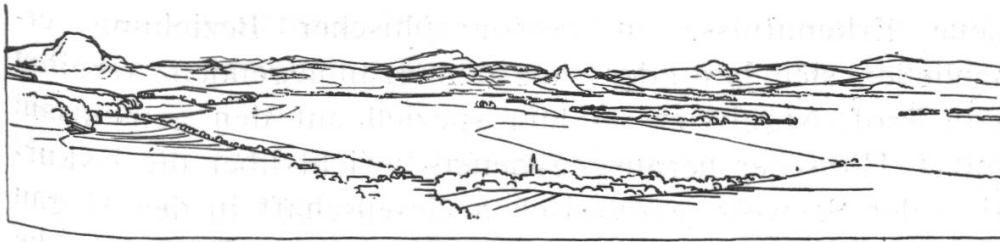
Das Hegauer Vulkangebiet, vom Friedinger Schloßchen gesehen (oder): von Osten gesehen.
