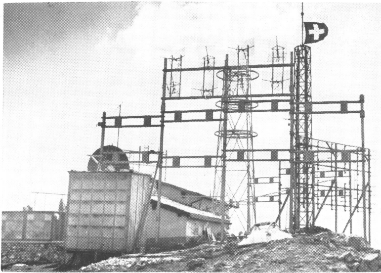
Die stark ausgebauten Relaisstation auf dem Chasseral, die im europäischen Fernsehverkehr eine wichtige Rolle zu spielen hat, bereit zum Empfang einer norwegischen Fernsehkommission, welche gegenwärtig schweizerische Fernseheinrichtungen studiert.
