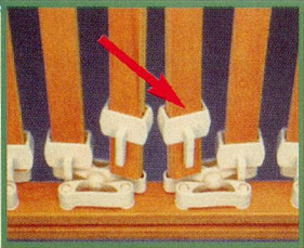
Patentierte Härteverstellung, 2 Punktlagerung
