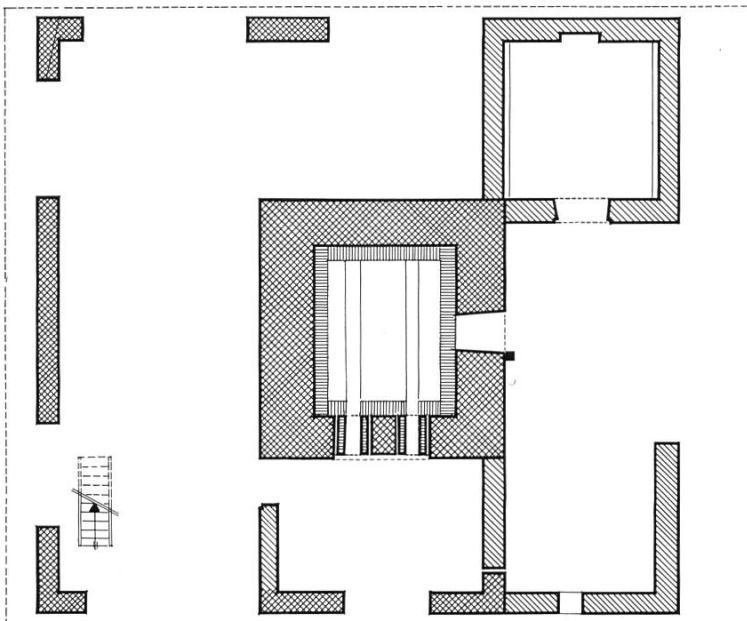
Abb. 7 Grundriss Erdgeschoss
