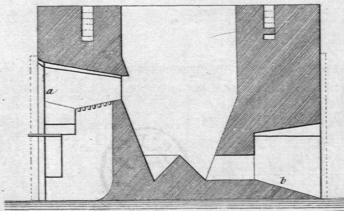
Durchschnitt nach C D.
