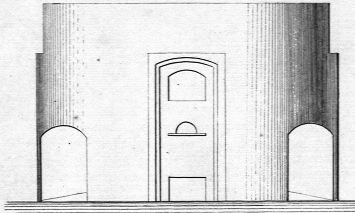
Vordere Ansicht des Kalkofens.
