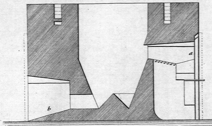
Durchschnitt des Ofens nach A B.
