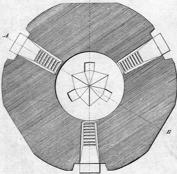
Grundriß der Roste.
