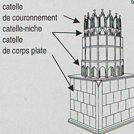
Poêle à tour gothique, 15 e siècle.
