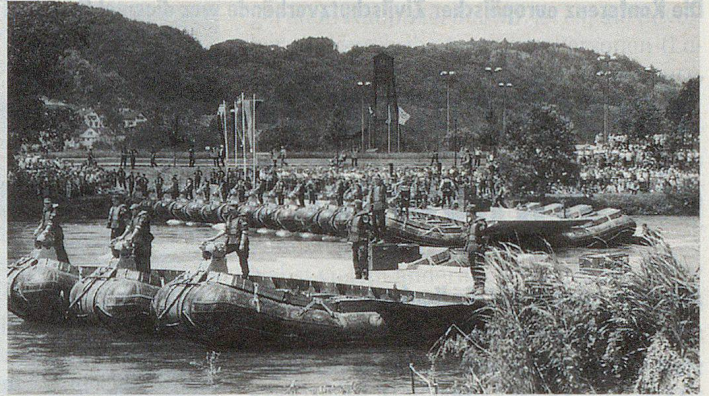
Die Schweizer fahren das letzte Anschlussstück ein.
