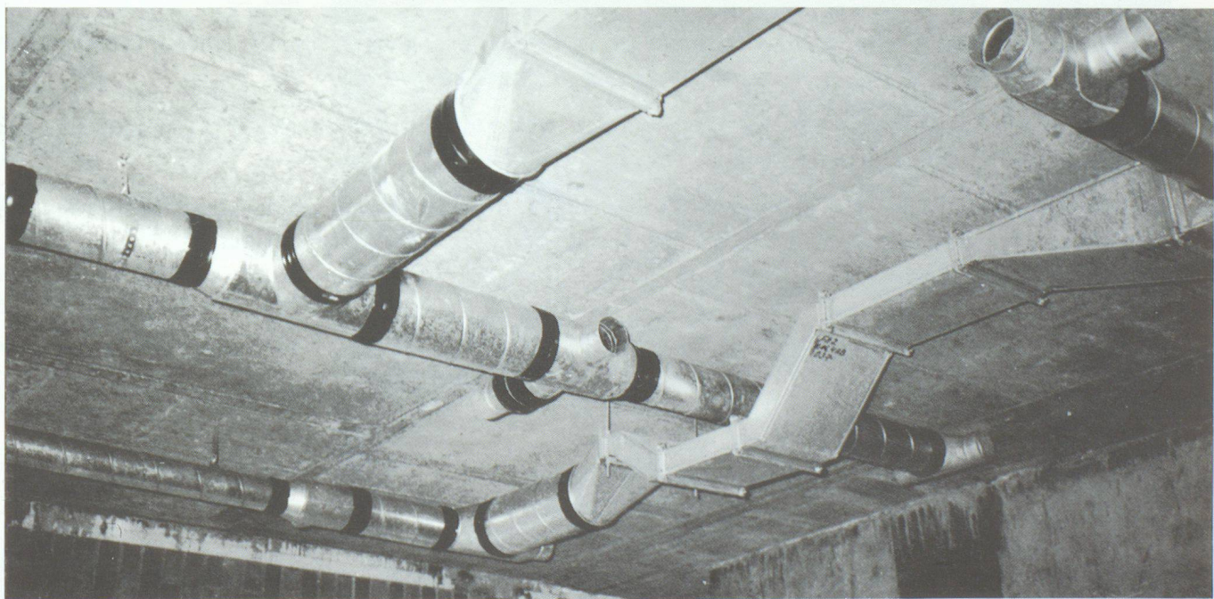
Übergang von Wickelfalz- auf Alu-Flex-Rohr.
