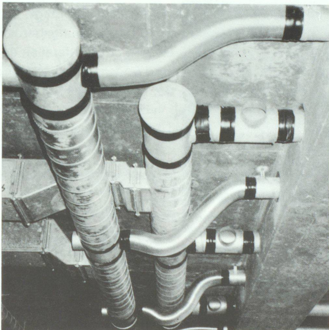
Übergang von Wickelfalz- auf Alu-Flex-Rohr.
