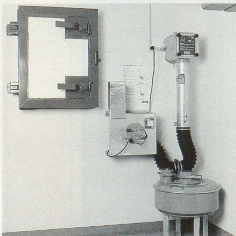
Schutzraum-Abschlüsse und -Belüftungs-Anlagen
