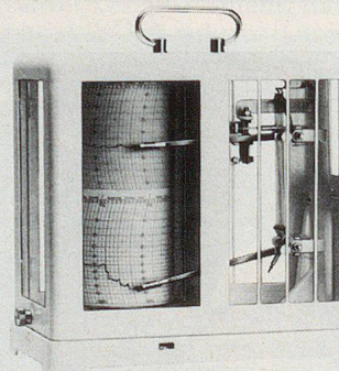
Abb.: Thermo-Hygrograph Typ 252 zur Registrierung von Temperatur und Feuchtigkeit
