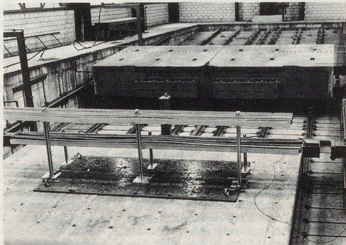
Schocktest-Anlage in Wimmis.
