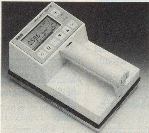
Kontaminationsmonitor Contamat FHT 111 M von FAG mit Nachweisempfindlichkeit und digitaler/analoger Messwertanzeige.
