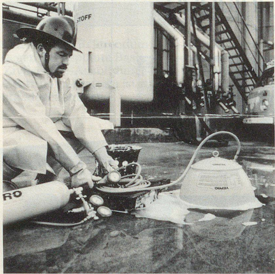
Dichtkissen-Einsatz
