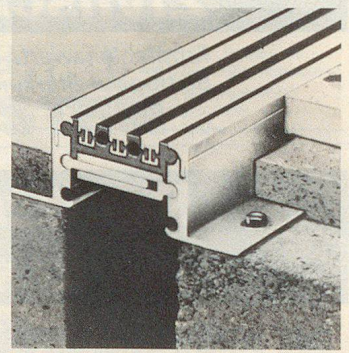
DEFLEX-Dehnfugenelement – mit diesen Dilatationsfugensystemen werden die äusserst schädlichen Schwundrisse bei befestigten Bauten und Anlagen vermieden.
