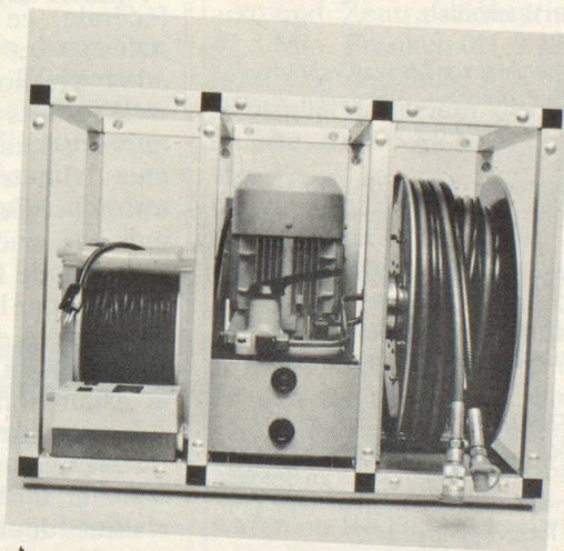
Antriebs-einheiten
