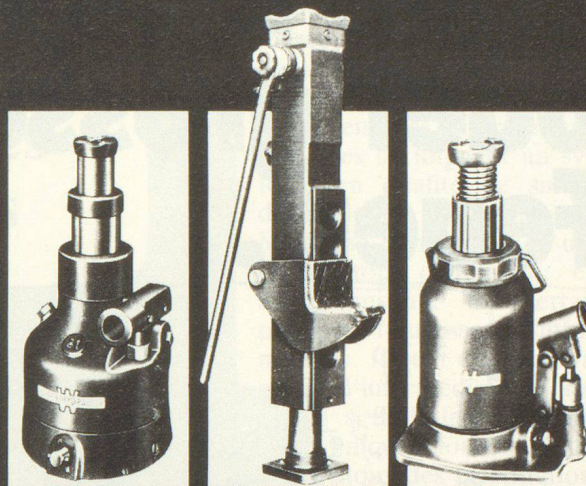
Typ „HV“ mit zwei Hubkolben, geschlossene Bauart von 2 - 12 t Hubkraft, 5 Modelle
