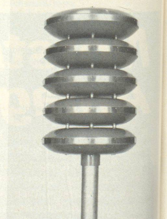
Mehrzweck-Tyfon, kombiniert für Zivilschutz, Wasser, Feuerwehr und KKW.
