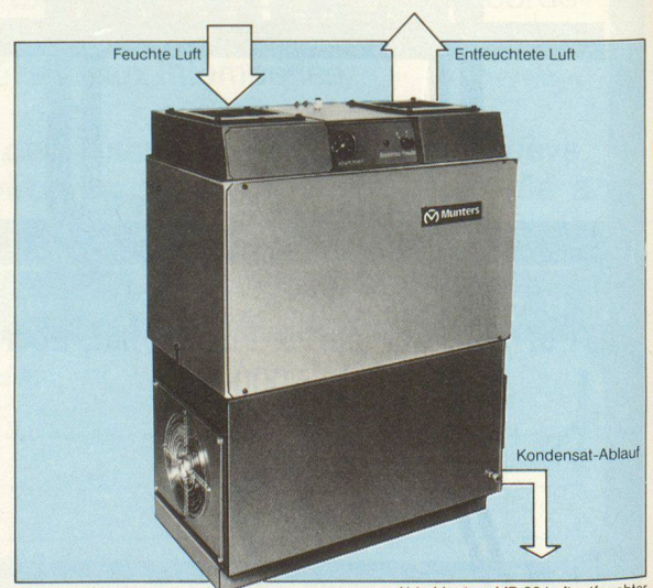
Abb. Munters MD 08 Luftentfeuchter
