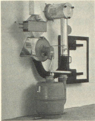
Schutzraumbelüftungsanlage mit Warmwasserluftheritzer.
