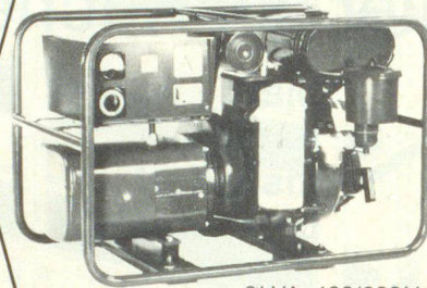
6 kVA - 400/230 V
