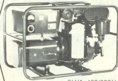
6 kVA - 400/230 V
