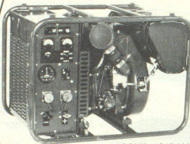
1200 W - 12/24 V
