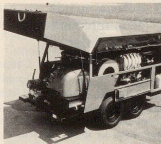
Tanklöschanhänger TSL 2000 ZS 2 mit Zivilschutzspritze Typ 2
