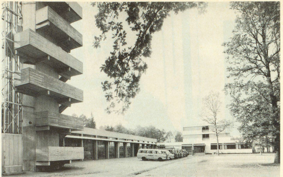
Im Hintergrund das Hauptgebäude der neuen Schule. In der Mitte die Garagen. Im Vordergrund der 26 m hohe Feuerwehrturm
