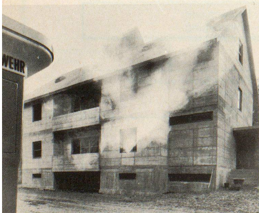
Ein ganz aus Stahlbeton gebautes grosses Brandhaus ermöglicht die realistische Ausbildung und die Simulation aller möglichen Gebäudebrände
