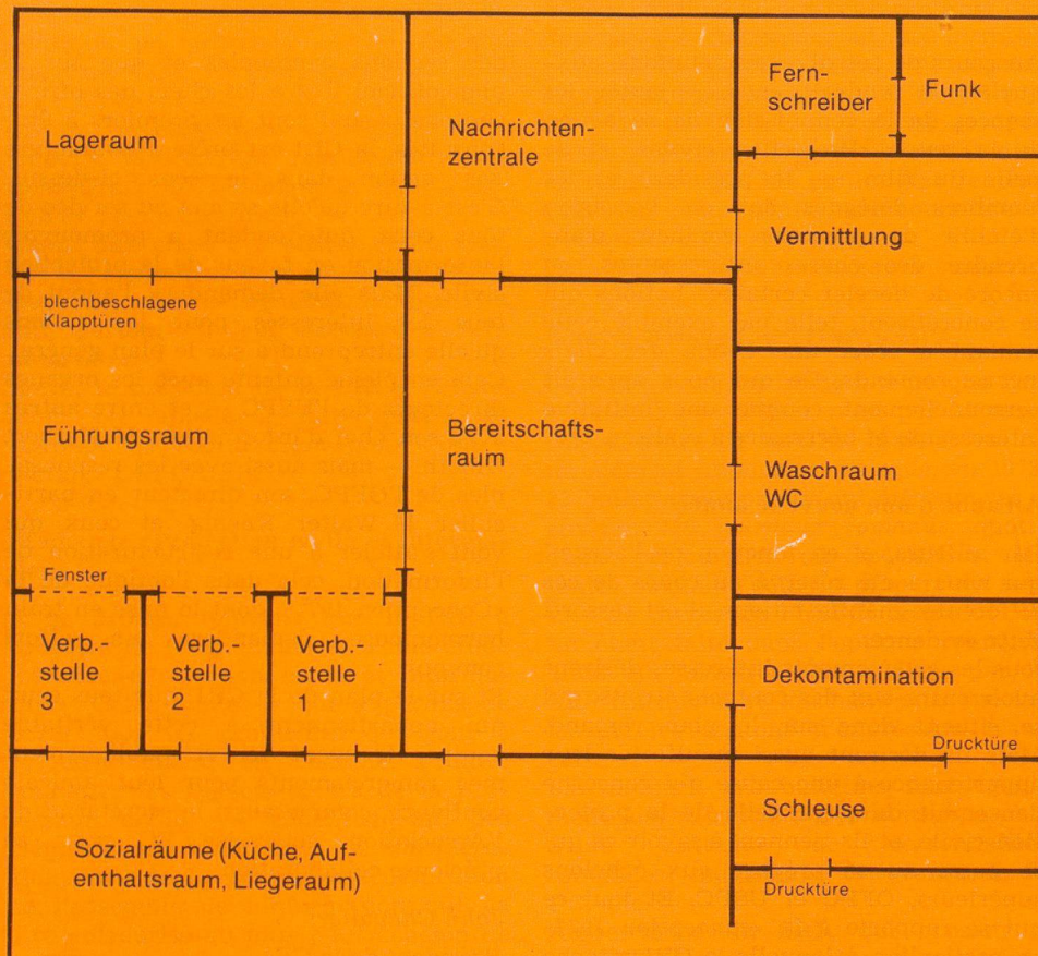
Schematische Darstellung der Katastrophenleitstelle
