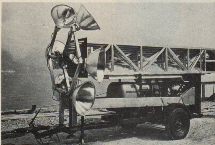
Fig. 34. Grande installation montée sur remorque
