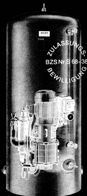
Druckkesselanlage
