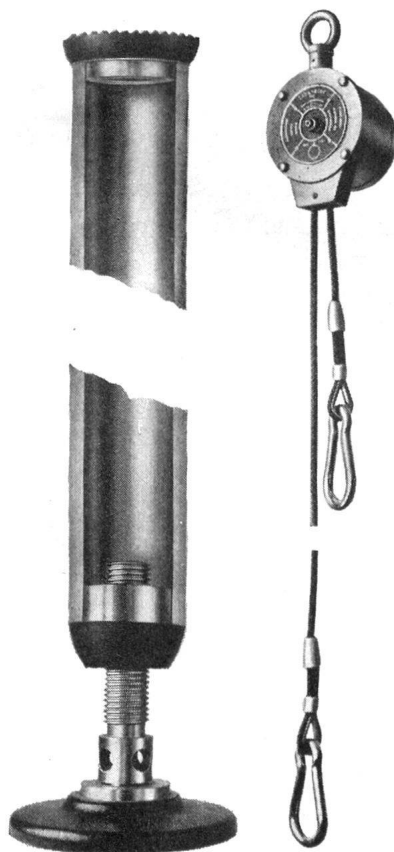
◀ «Meili-Liberator» zur Rettung aus brennenden Gebäuden und Hochhäusern. Geräte für jede Seillänge bis 250m und darüber. Keine Seiltrommel, daher sehr leicht und handlich. Prospekt 98
