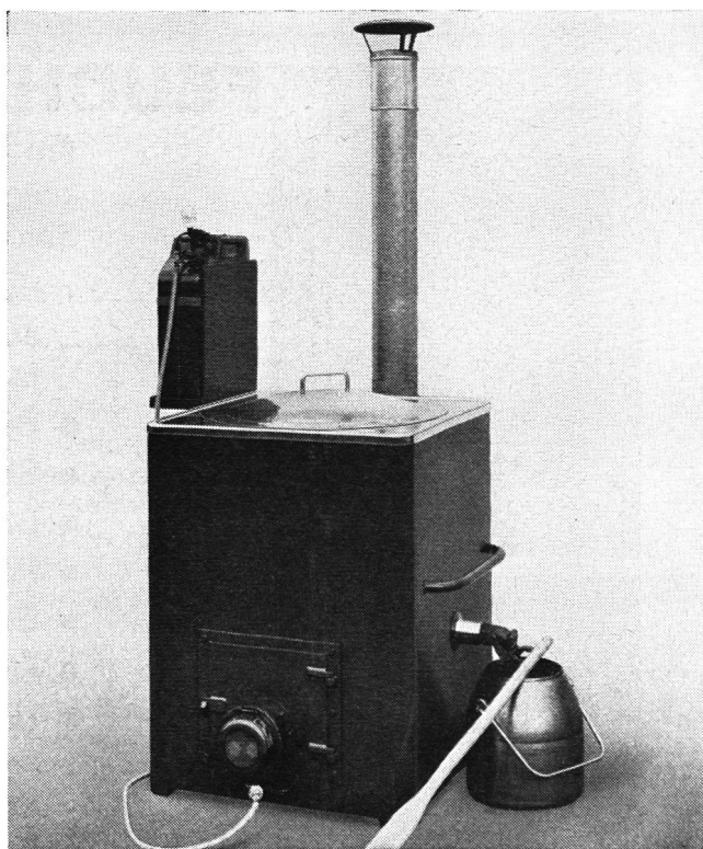
Kochkessel 150 Liter mit losen Deckel. Feuerung mit flüssigen oder festen Brennstoffen.
