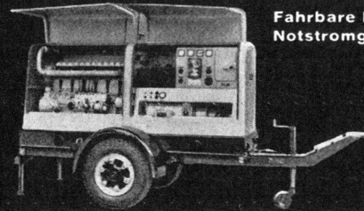
Vollautomatische Diesel- Notstromgruppe, 100 kW
