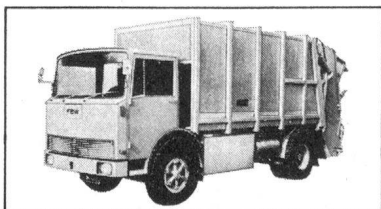
2) FBW: L 35 U Kehrrichtwagen Motor: FBW - CUA (130 PS) Getriebe: Allison MT-41 (Automat)
