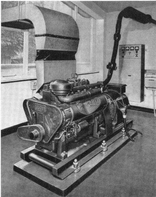
LISTER — Deselektische Anlage mit Netzausfall-Vollautomatik, 57,5 kVA, luftgekühlt
