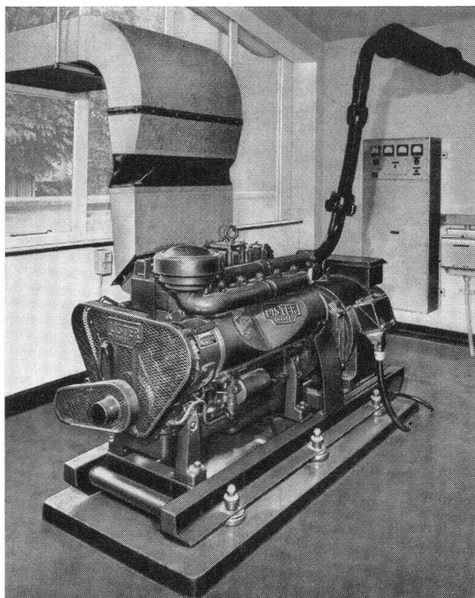
LISTER — Deselelektrische Anlage mit Netzausfall-Vollautomatik, 57,5 kVA, luftgekühlt
