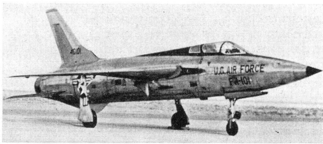
Republic F-105 «Thunderchief» nach einem Probeflug im USAF-Erprobungszentrum Edwards bei Muroc (Kalifornien). Das in diesem Jagdbomber eingebaute Triebwerk ist eine Strahltriebchine Pratt & Whitney mit einer Maximalschubleistung von 6800 kg.
